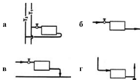
Рис. 2.4 Схемы разностороннего присоединения труб к радиаторам при движении теплоносителя сверху вниз: а, б – при числе секций в радиаторе более 27 (в насосных системах) и более 16 (в гравитационных системах); в, г – в обратную магистраль под радиатором и над радиатором
