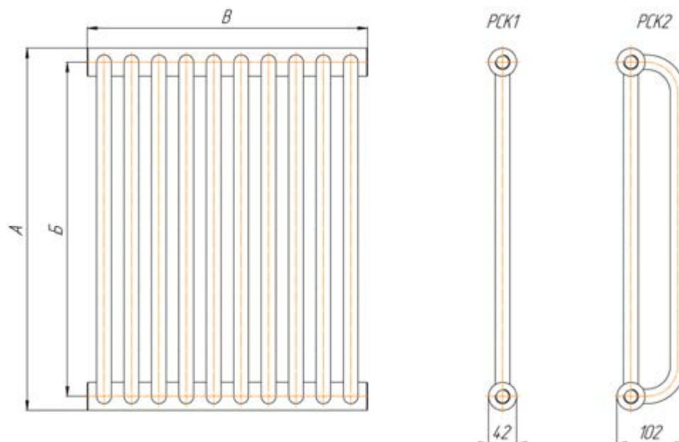
Рис. 1.2 Модификации радиаторов «PSK».
