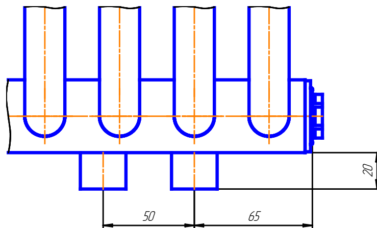
Рис. 1.4 Узел нижнего подключения. Присоединительная резьба – внутренняя 1/2".
